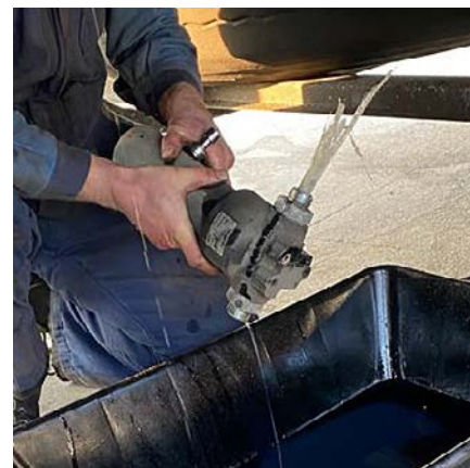
Resten van filtermateriaal in het hydrauliek systeem
